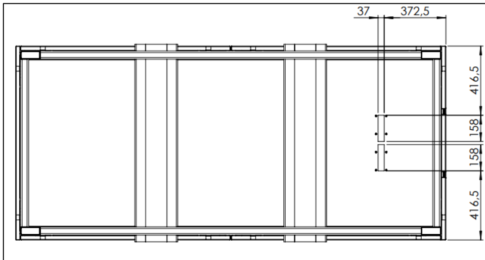
Abbildung 16: Kabeleinführung von unten
