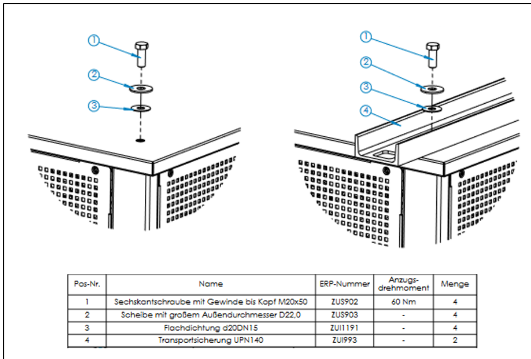
Abbildung 10. Demontage Transporttraverse
