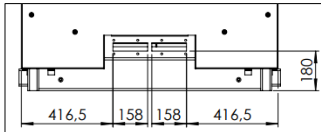
Abbildung 15: Kabeleinführung von vorne
