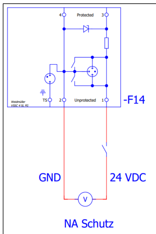
Abbildung 26: Anschlussbeispiel Kuppelschalter – AA1, AA2
