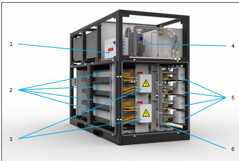
Abbildung 7: Komponenten hinten
