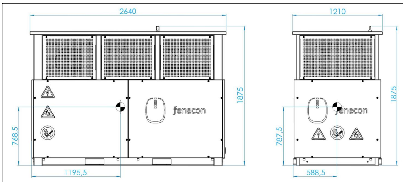
Abbildung 1: Stromspeicher mit Bemaßung (Toleranz Schwerpunkt +/- 50 mm) [in mm]
