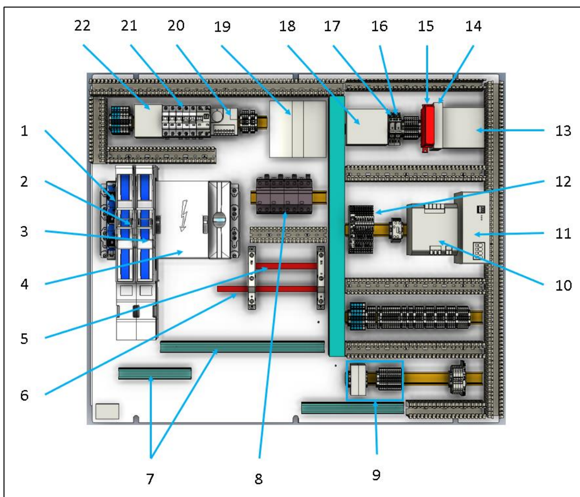
Abbildung 9: Komponenten control cabinet (AA3)
