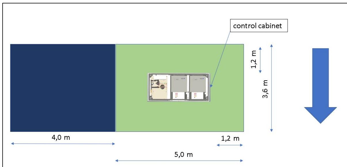
Abbildung 12: Aufstellungskonzept – Platzbedarf
