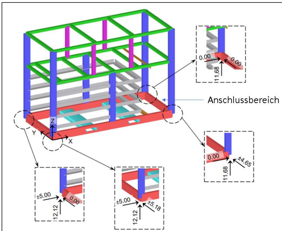
Abbildung 13: Lastabtragungspunkte (Einheit: kN)
