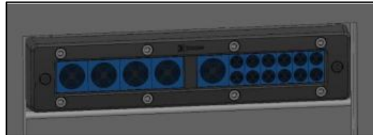
Abbildung 14: Kabeleinführung - Roxtec
