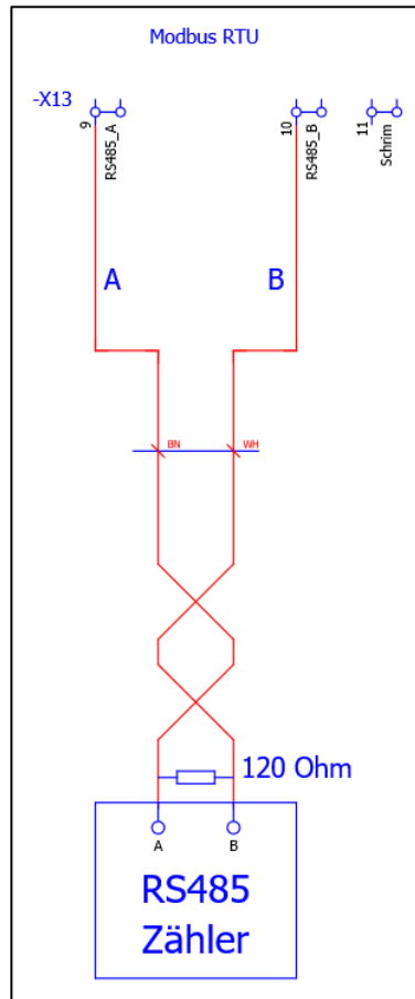
Abbildung 24: Anschlussbeispiel RS485-Schnittstelle – AA3
