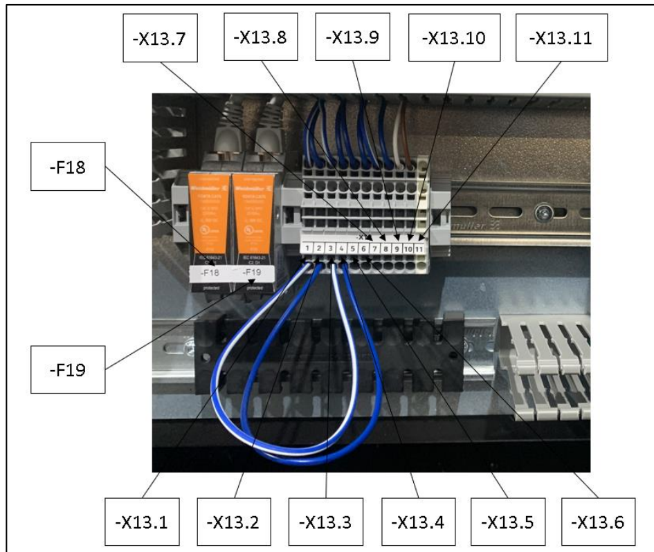
Abbildung 23: Anschluss Kommunikation und Signale – AA3
