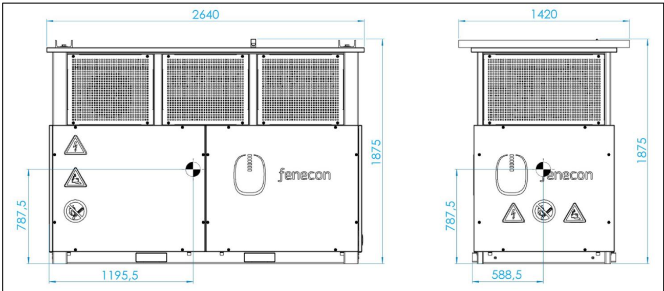
Abbildung 2: Transportmaße, Stromspeicher mit Transporttraversen (Toleranz Schwerpunkt +/- 50 mm) [in mm]
