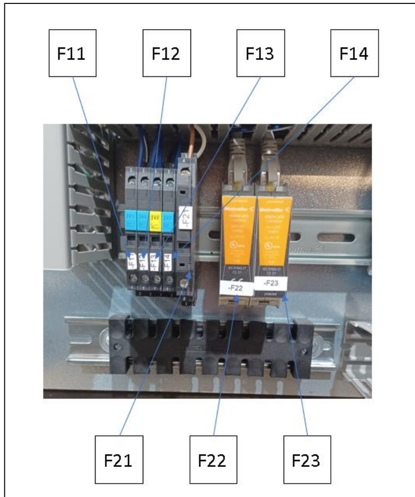
Abbildung 21: Anschluss Kommunikation und Signale – AA1, AA2
