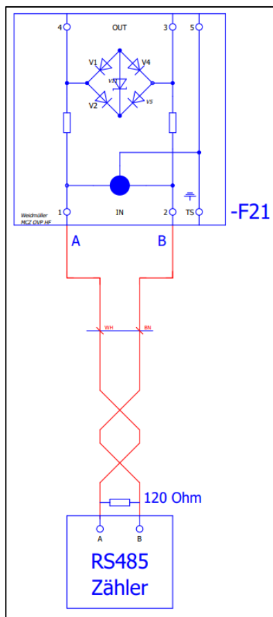
Abbildung 22: Anschlussbeispiel RS485-Schnittstelle – AA1, AA2
