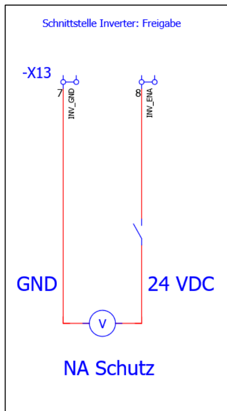
Abbildung 28: Anschlussbeispiel Kuppelschalter - AA3
