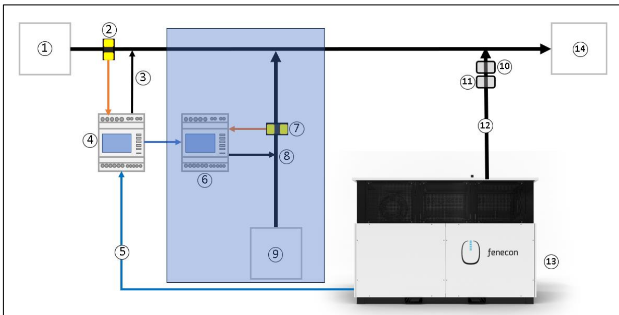
Abbildung 17: Single Line Diagramm - Standardaufbau des Systems
