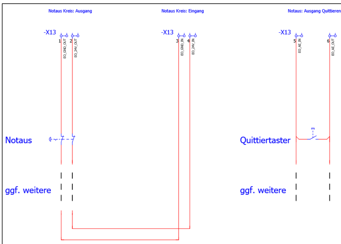
Abbildung 27: Anschlussbeispiel externer Not-Halt und Quittiertaster -AA3
