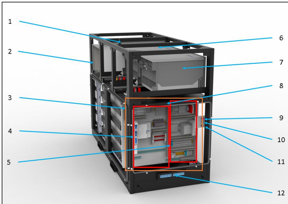
Abbildung 6: Komponenten vorne
