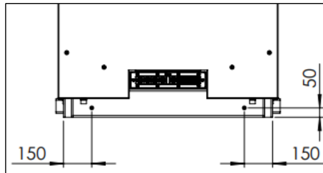
Abbildung 20: Erdungsanschluss vorne
