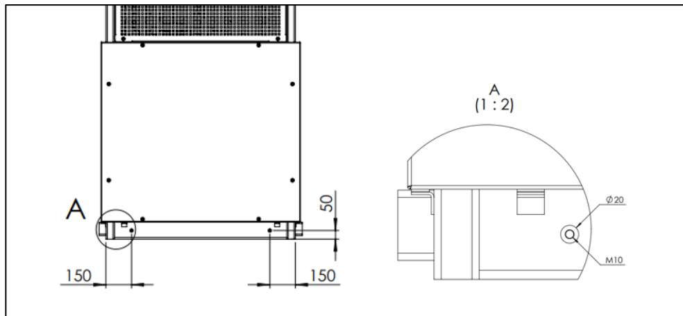
Abbildung 19: Erdungsanschluss hinten
