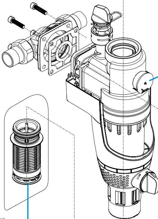
Ersatzfilterelement YSK233200909
