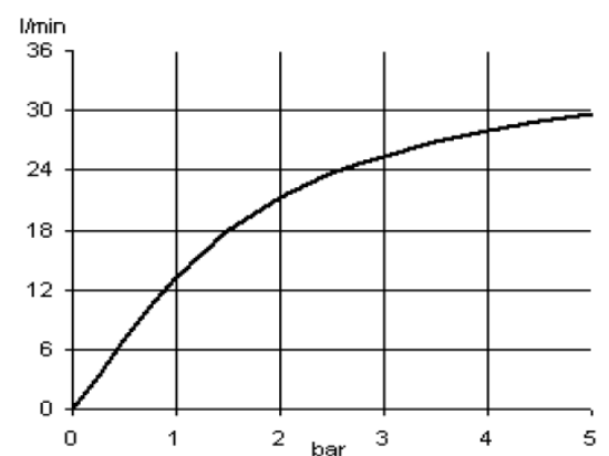
Durchflussdiagramm
