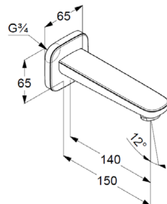
Maßzeichnung
