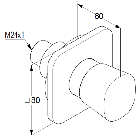
Maßzeichnung/ Dimensional drawing
