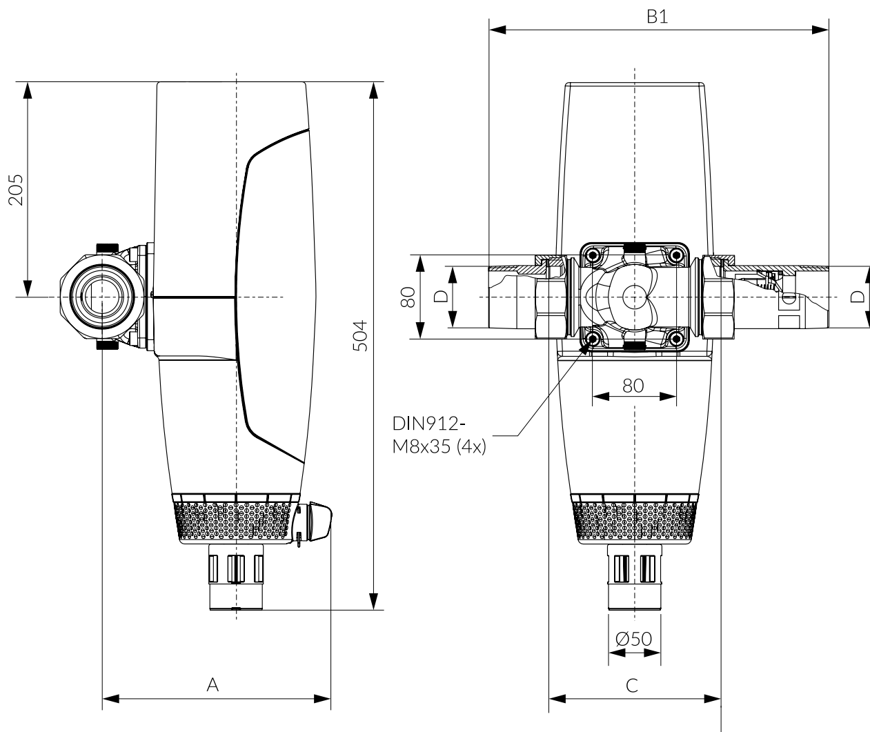
Maße / dimensions [mm]
