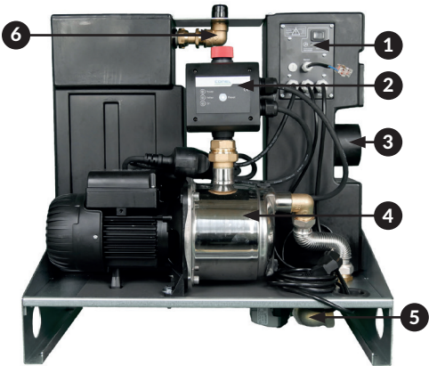
Abb. 4.2.1 Conel Flow Regen-Meister Baugruppe
