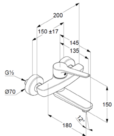
Maßzeichnung
