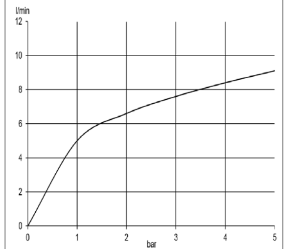
Durchflussdiagramm
