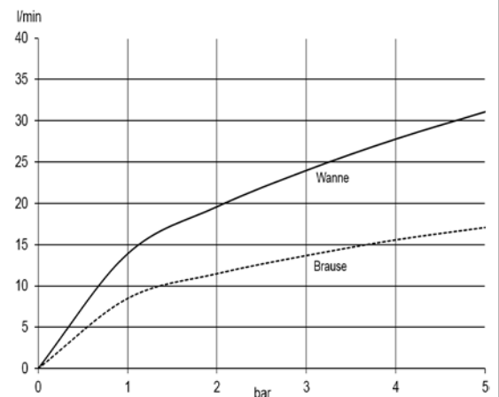
Durchflussdiagramm
