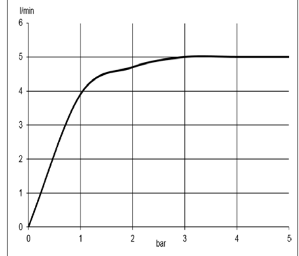
Durchflussdiagramm
