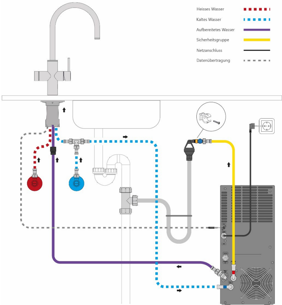
Abbildung 5: Installationschema
