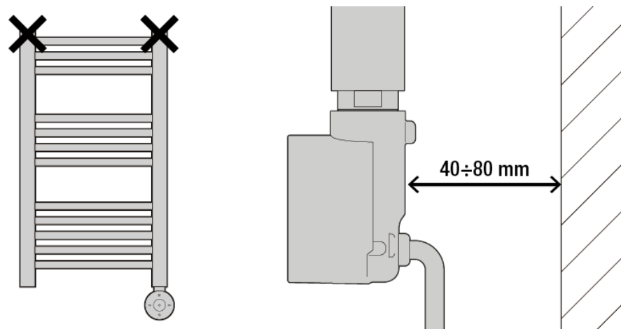
Abbildung 5 Position des -Reglers
