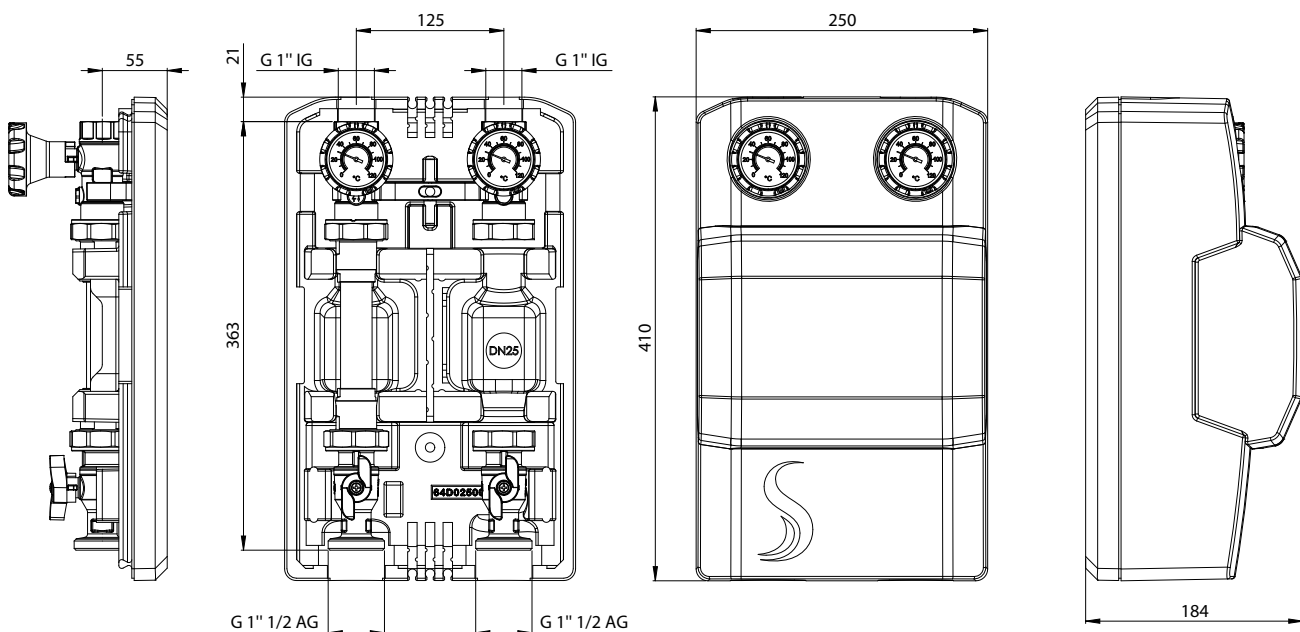
Maßzeichnung Pumpengruppe DN 25
