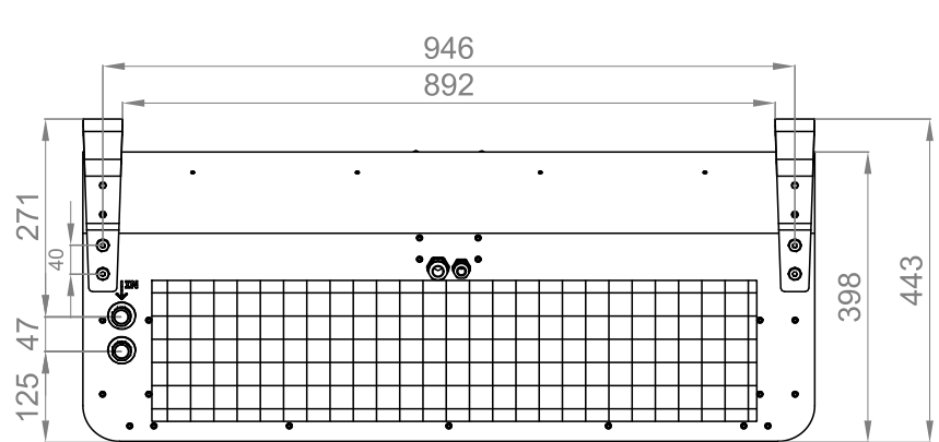
Unteransicht
