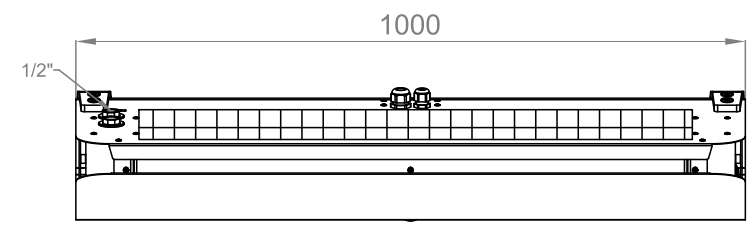
Rückansicht
