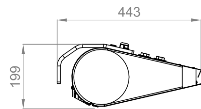
Seitenansicht
