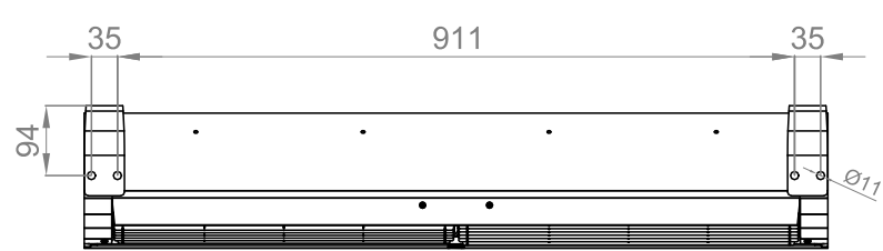
Rückansicht
