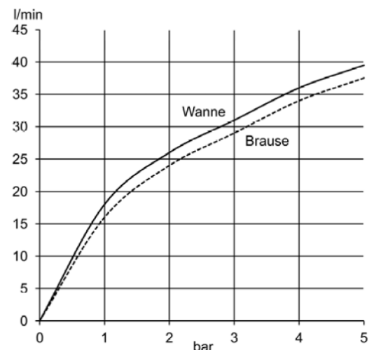
Durchflussdiagramm
