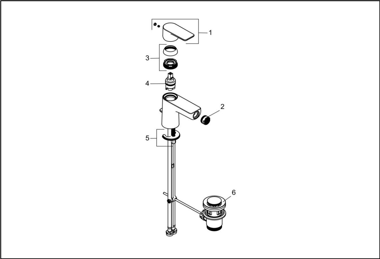
V3DEBDSM Einhand-Bidetbatterie derby V3 Single-lever bidet mixer derby V3 mit Ablaufgarnitur schwarz matt VIGOUR with drain set matt black VIGOUR
