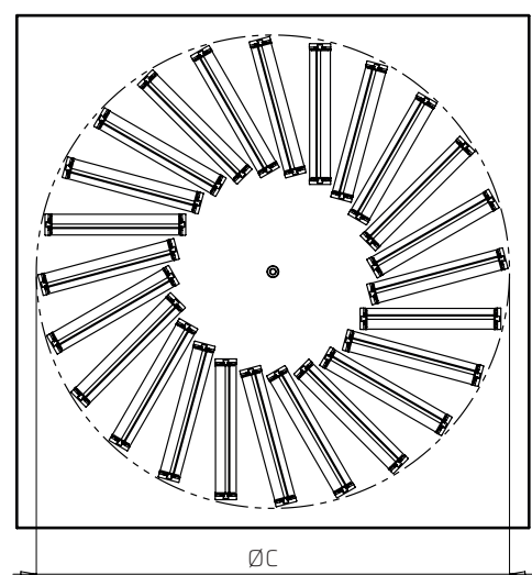
Rückansicht
