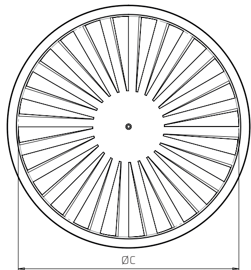
Rückansicht
