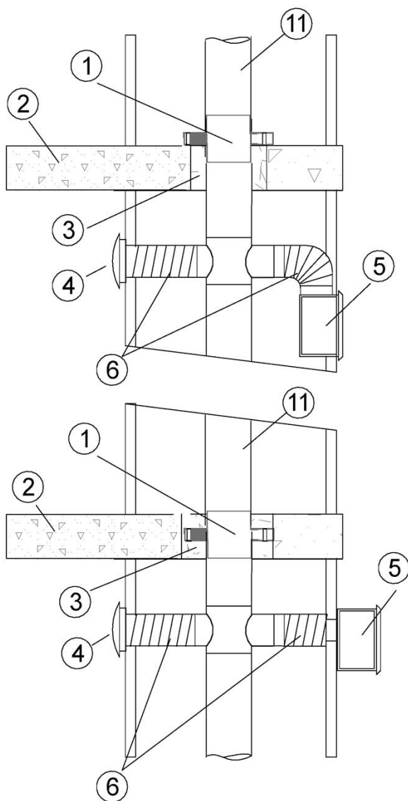
Einbausituation mit Zentralventilationsanlage
