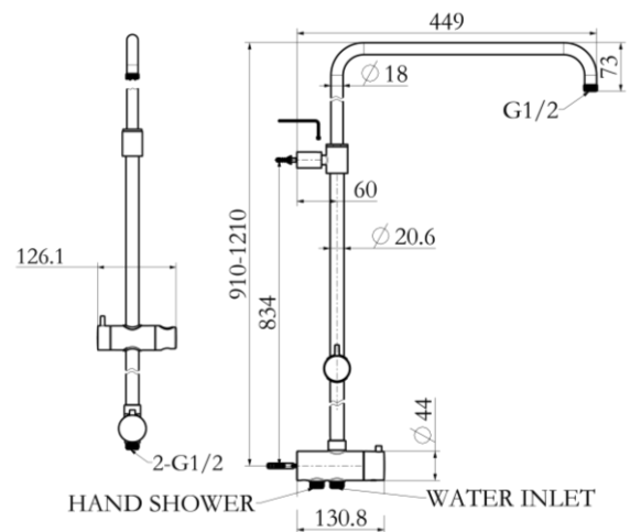
Maßzeichnung
