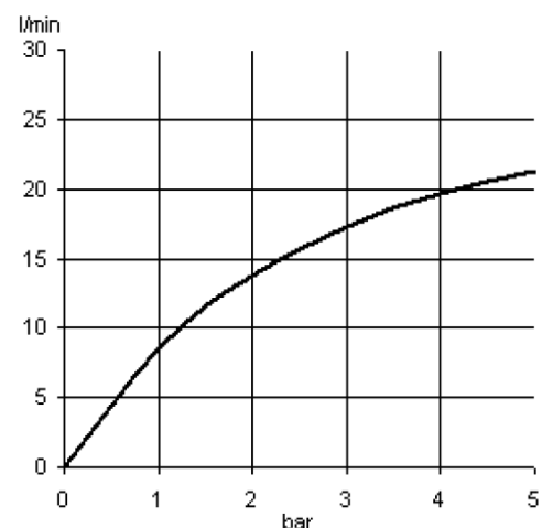
Durchflussdiagramm
