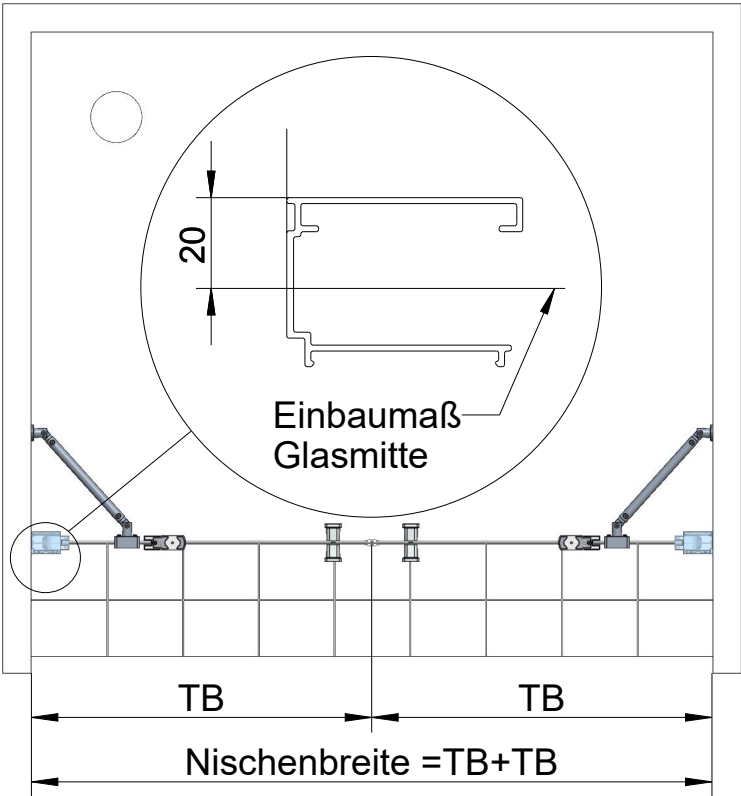
Auslieferungszustand
