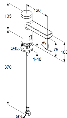
Maßzeichnung/ Dimensional drawing
