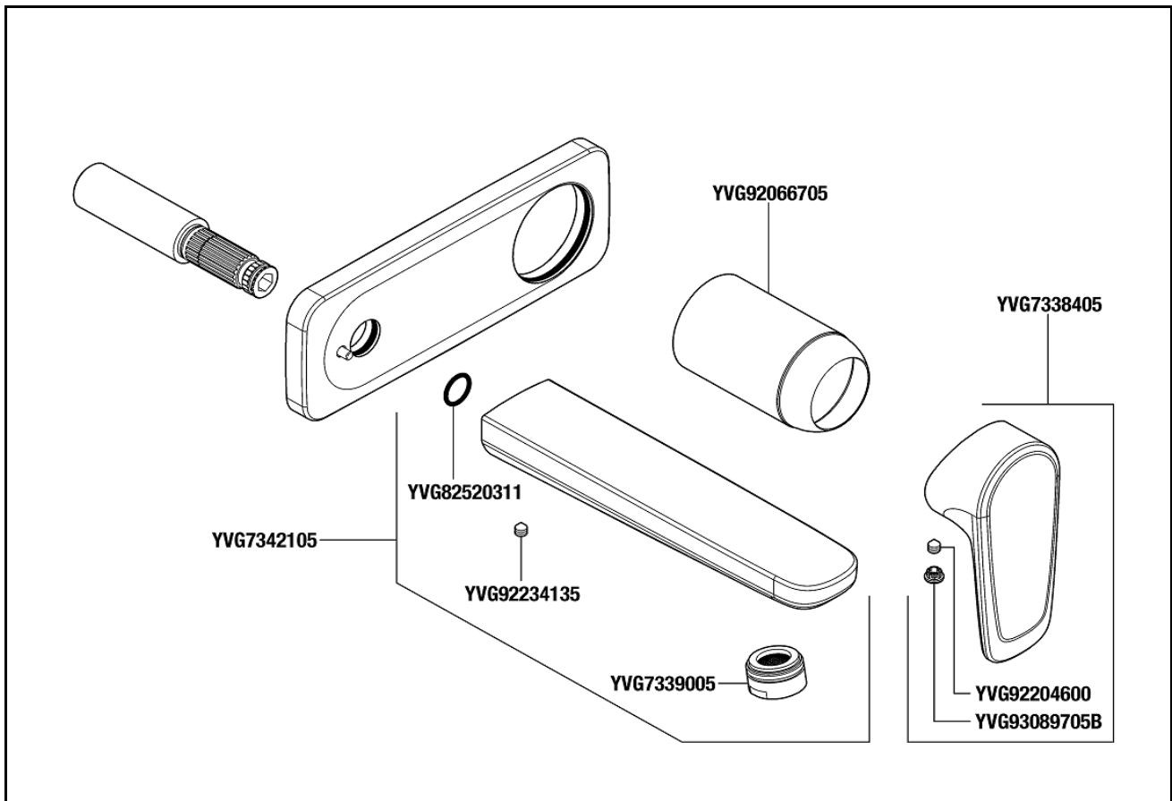
DESFWW180 Farbset Wascht.-Wandarmatur derby style für DEUPKWW Auslauf 180mm verchromt VIG. Finish set wall mounted m. derby style for DEUPKWW Spout 180mm chromed VIG.
