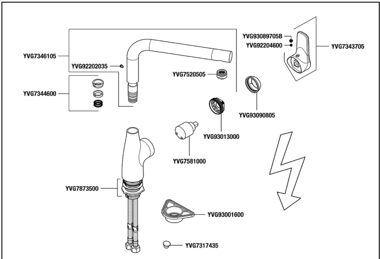
DESSPNDL Einhand-ND-Spültischbatterie derby style Single lever LP sink mixer derby style m. L-Auslauf schwenkbar verchromt VIGOUR with L-spout slewable chromed VIGOUR
