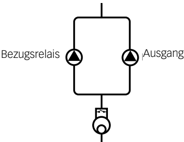
Beispielschema für Zwillingspumpen im solaren Vorlauf mit vorgelagertem Volumenmessteil
