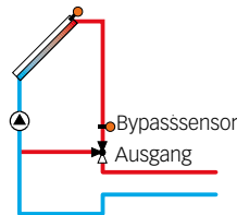
Beispielschemata für die verschiedenen Bypass-Varianten
