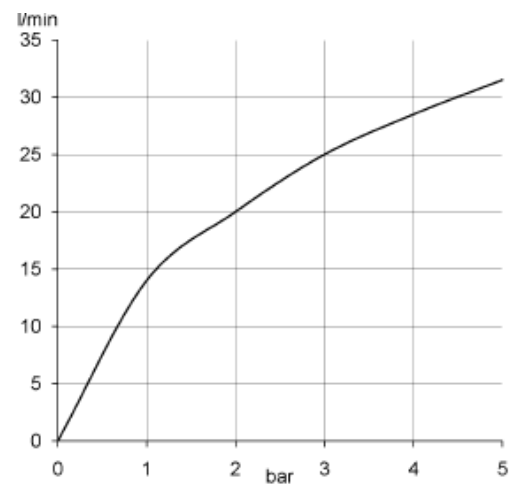
Durchflussdiagramm
