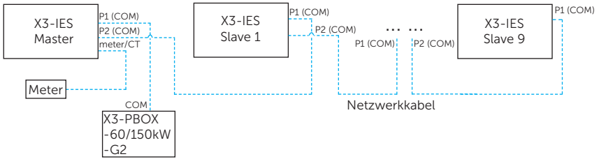
Parallelschaltung Methode 1:
