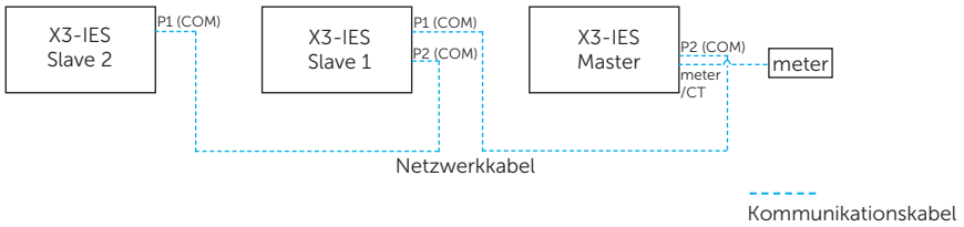
Parallelschaltung Methode 2:
