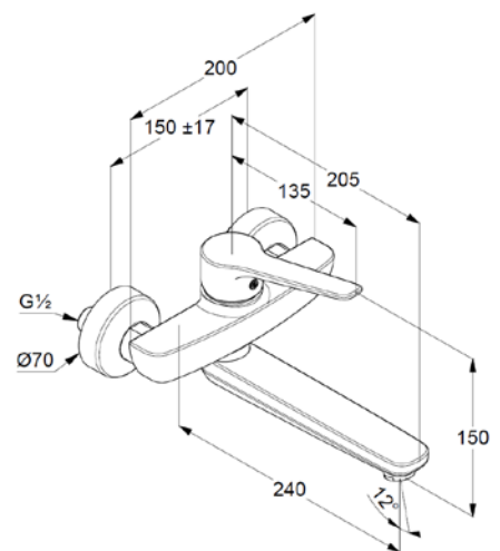
Maßzeichnung
