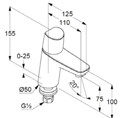
Maßzeichnung
