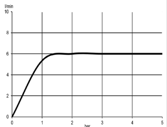
Durchflussdiagramm
