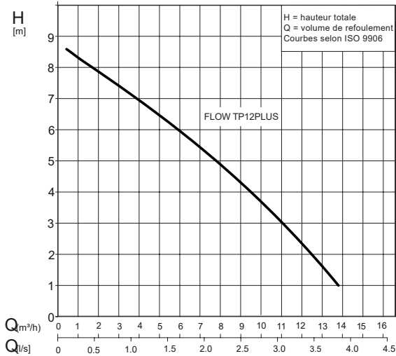
Courbe de performance 50 Hz
