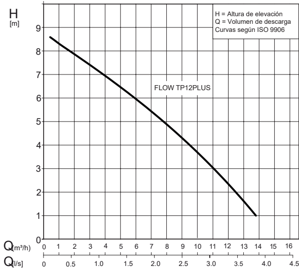
Curva de rendimiento 50 Hz
