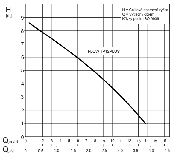
Výkonnostní křivka 50 Hz
