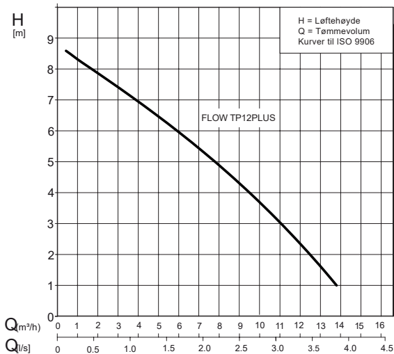
Ytelseskurve 50 Hz
