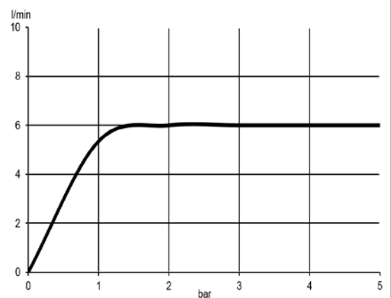
Durchflussdiagramm
