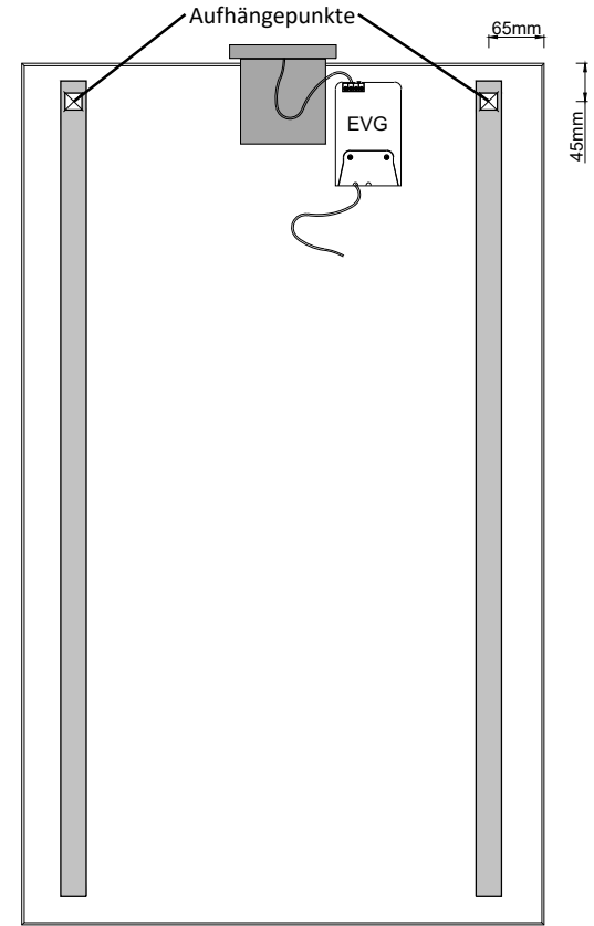
Rückansicht
