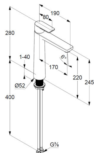
Maßzeichnung
