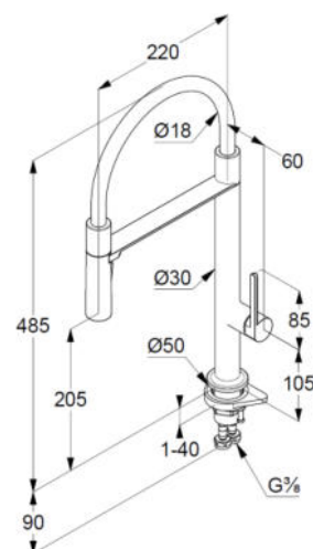
Maßzeichnung
