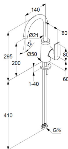
Maßzeichnung
