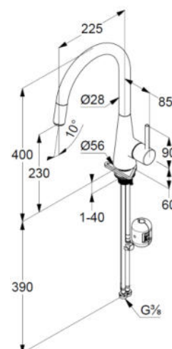
Maßzeichnung
