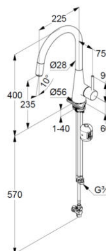
Maßzeichnung
