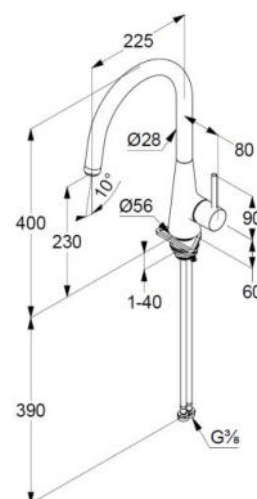
Maßzeichnung
