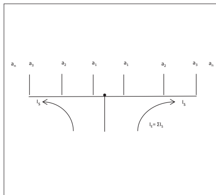
Einspeisung im Verlauf der Schiene oder Mittleinspeisung
