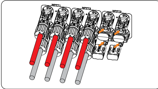
Abbildung 7-22 PV staubdichte Schnallen installieren
