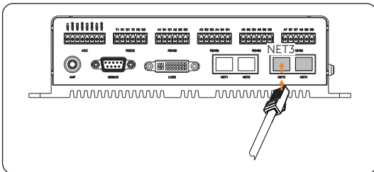
Abbildung 9-22 Ethernet-Kabel einstecken
