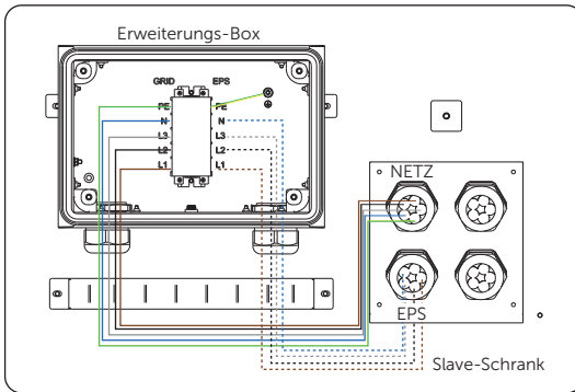
Abbildung 14-79 Schaltplan
