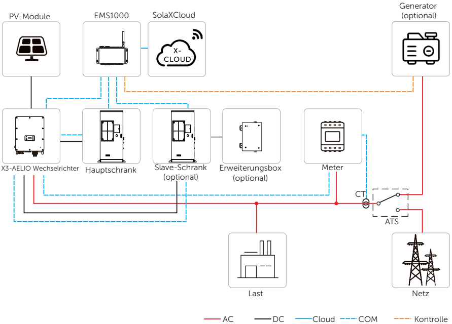
Abbildung 2-1 Systemübersichtdiagramm
