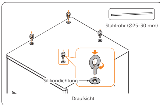
Abbildung 6-5 Ringschrauben anziehen
