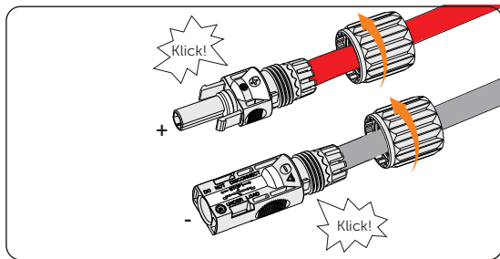
Abbildung 7-18 PV-Kabel sichern
