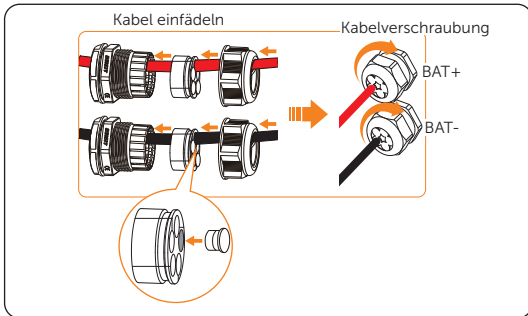
Abbildung 14-40 Stromkabel einfädeln
