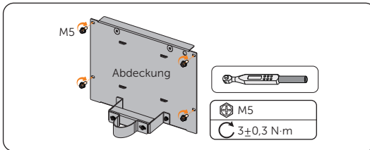
Abbildung 14-45 Abdeckung wieder anbringen
