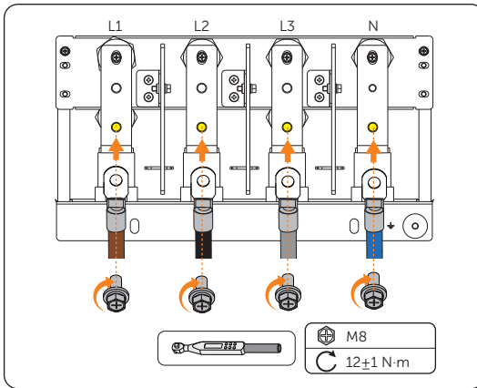
Abbildung 14-56 M8-Schrauben anziehen
