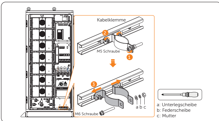
Abbildung 7-74 M6-Schrauben herausdrehen
