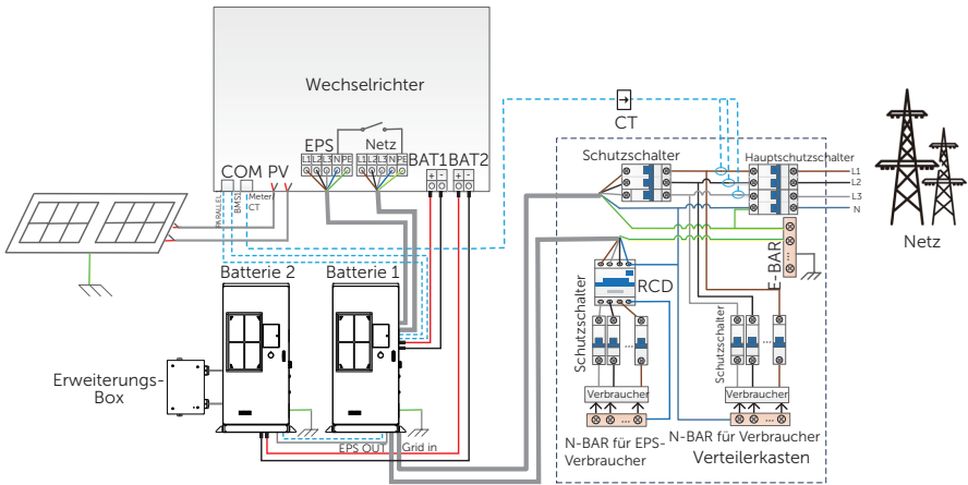
Abbildung 2-34 Partielles Verbraucher-Backup für Australien
