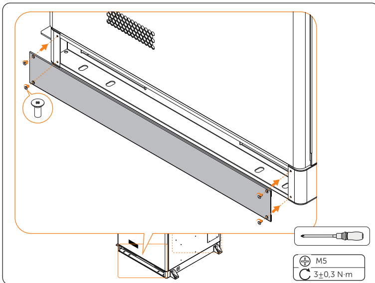
Abbildung 6-15 Abdeckungen befestigen
