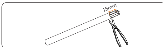
Abbildung 9-19 Kabelmantel abisolieren
