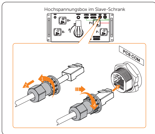
Abbildung 14-67 Kommunikationskabel einstecken
