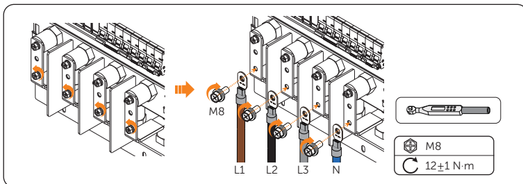
Abbildung 7-78 L1/L2/L3/N-Drähte anschließen
