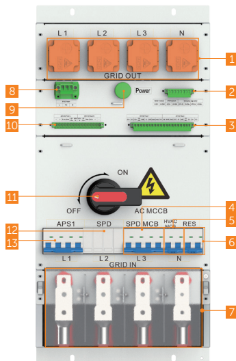
Abbildung 2-10 Frontplatte
