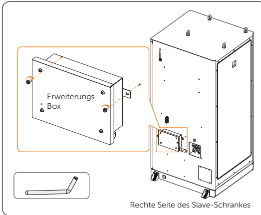
Abbildung 14-73 Erweiterungsbox installieren
