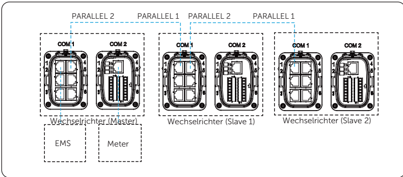
Abbildung 14-92 Kommunikationsdraht
