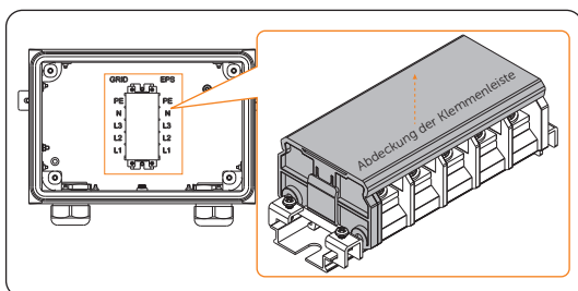
Abbildung 14-76 Abdeckung öffnen
