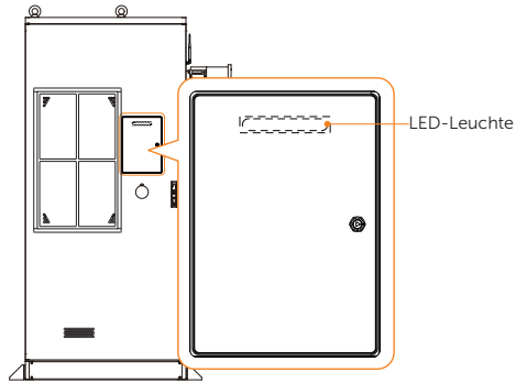
Abbildung 2-21 LED-Leuchte
