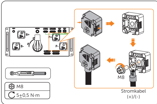
Abbildung 14-44 Stromkabel anschließen
