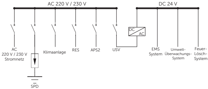
Abbildung 2-36 Elektrisches Blockdiagramm
