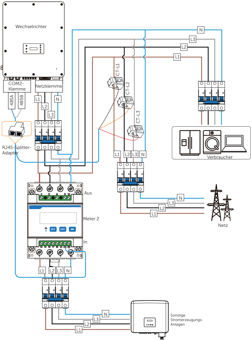
Abbildung 14-25 Anschlussplan von CT und direkt angeschlossenem Meter
