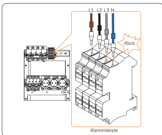
Abbildung 14-47 Stromkabel einstecken
