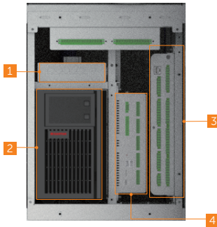
Abbildung 2-6 Teile-Beschreibung (Kontrollbereich)
