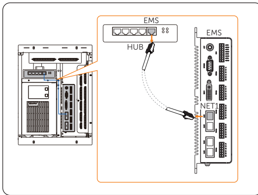
Abbildung 14-103 Kabel ausziehen
