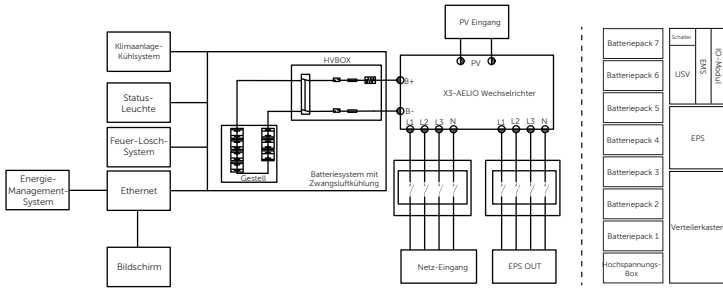
Schaltplan der AC-Hilfsstromversorgung
