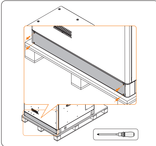
Abbildung 6-1 Abdeckung entfernen
