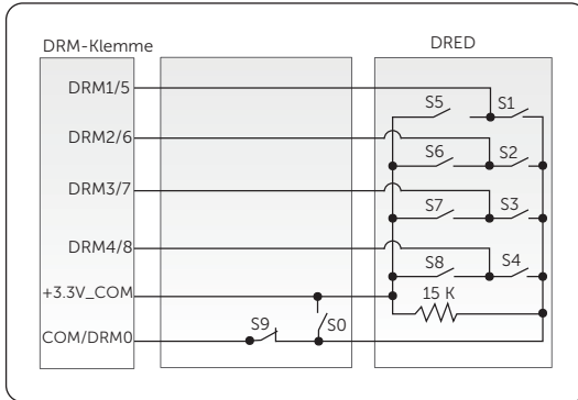
Abbildung 7-42 DRED-Anschlussplan
