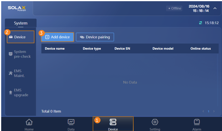
Abbildung 9-11 Geräte hinzufügen
