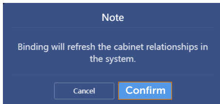
Abbildung 14-112 Kopplung bestätigen
