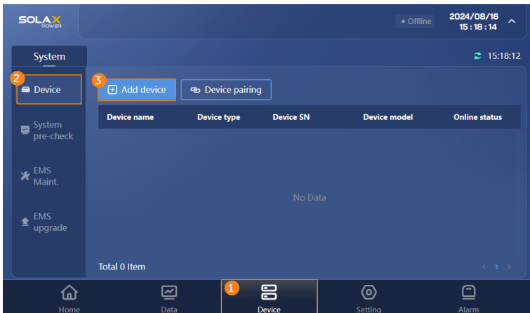
Abbildung 14-108 Geräte hinzufügen
