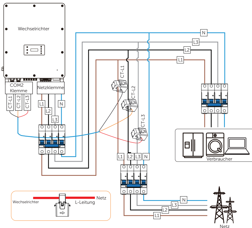
Abbildung 14-11 Systemverdrahtung mit CT
