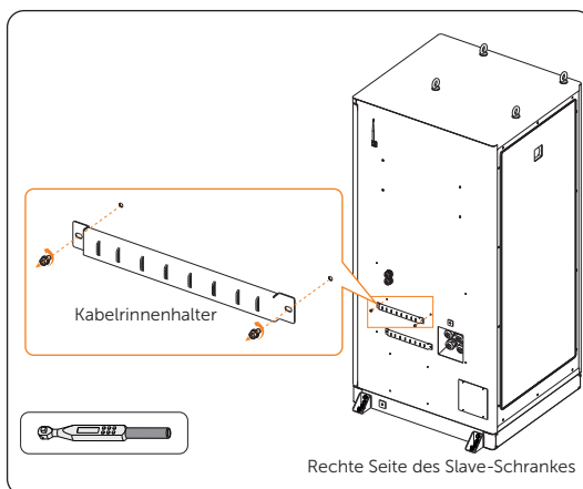
Abbildung 14-72 Kabelbinderhalterung entfernen
