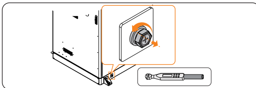
Abbildung 7-5 M12-Schraube abschrauben
