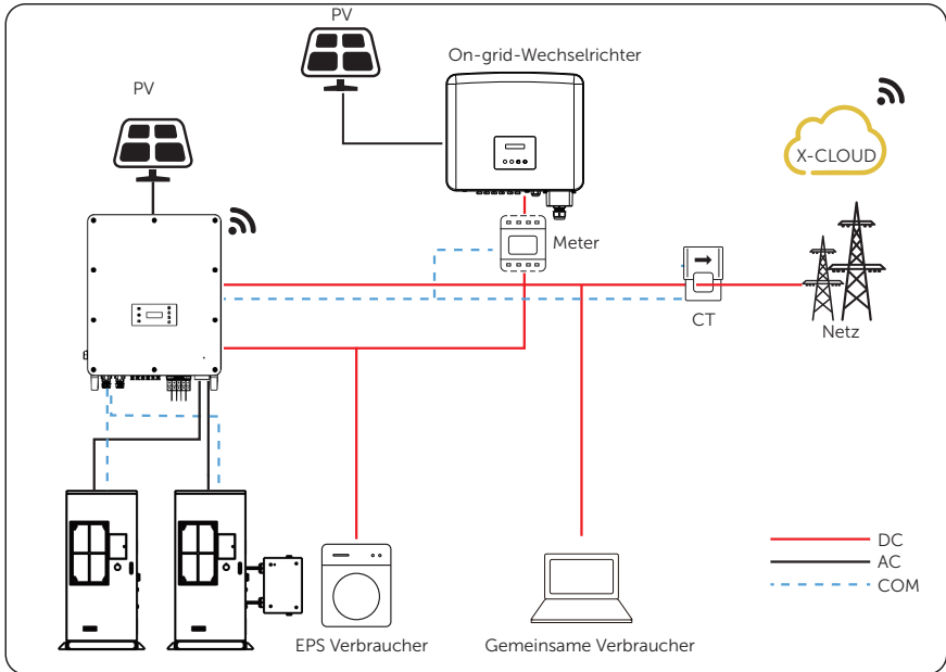
Abbildung 14-7 Anschluss an das Mikronetz
