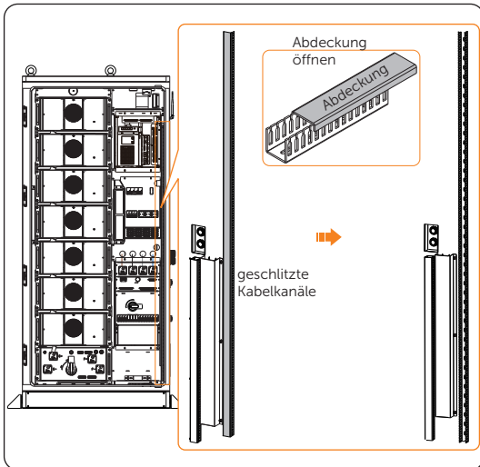
Abbildung 14-62 Abdeckungen öffnen
