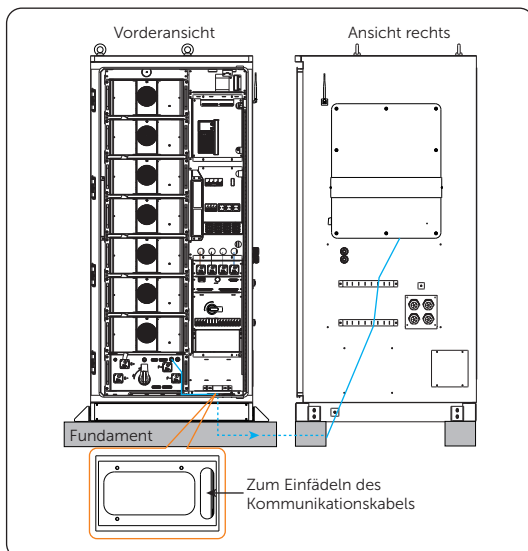
Abbildung 14-68 Kommunikationskabel einfädeln
