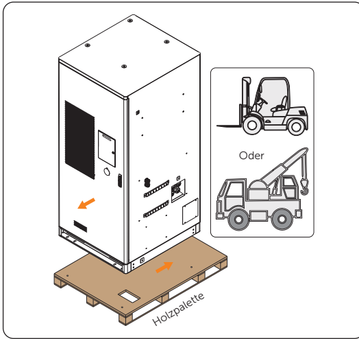
Abbildung 6-3 Schrank entfernen
