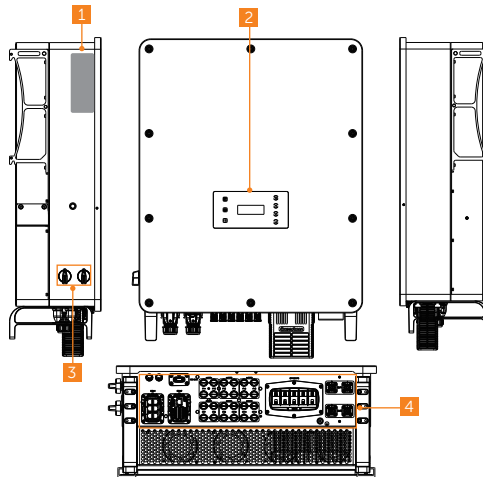
Abbildung 2-4 Teile-Beschreibung
