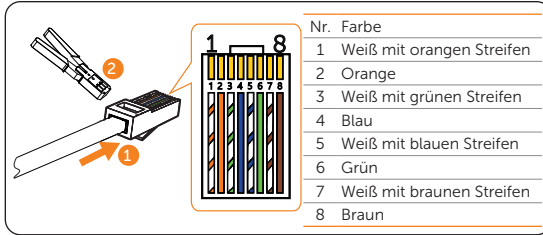
Abbildung 14-94 RJ45 crimpen
