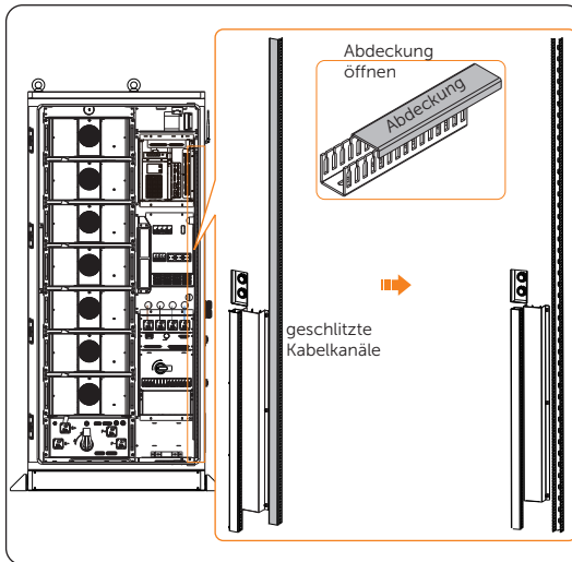
Abbildung 9-23 Abdeckungen öffnen
