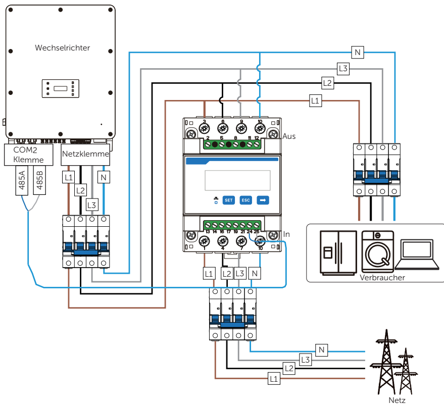
Abbildung 14-15 Systemverkabelung mit direkt angeschlossenen Meter
