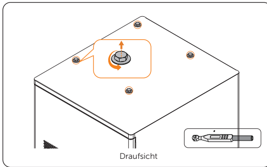
Abbildung 6-4 M20-Schrauben herausdrehen
