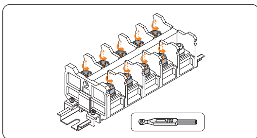
Abbildung 14-77 M5-Schrauben herausdrehen
