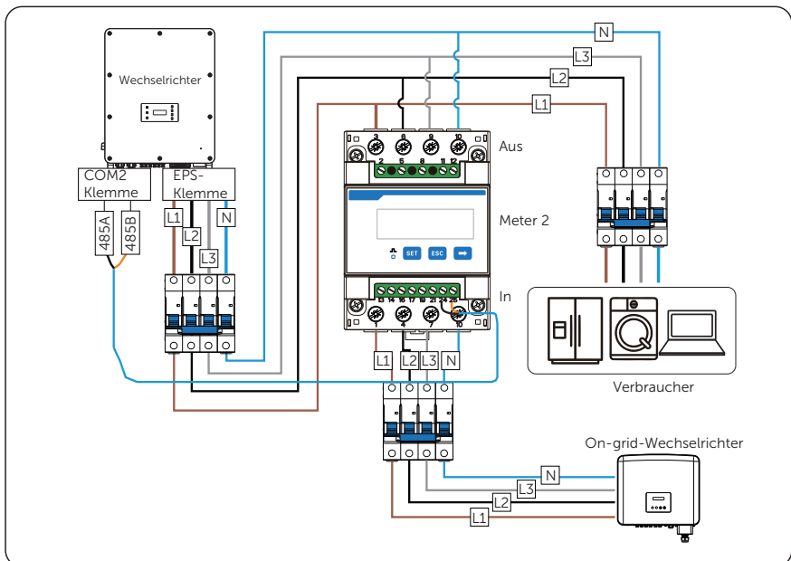
Abbildung 14-10 Anschlussplan von Meter an der EPS-Klemme
