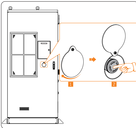
Abbildung 11-11 Not-Aus-Taste drücken
