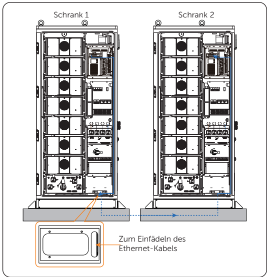
Abbildung 14-99 Ethernet-Kabel einfädeln
