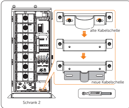
Abbildung 14-52 Klammer öffnen
