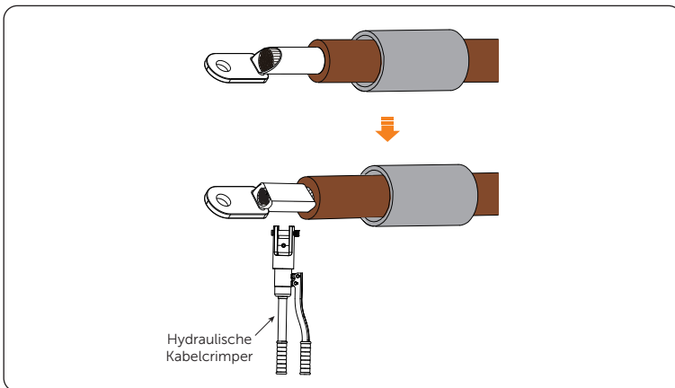
Abbildung 7-59 Crimpen
