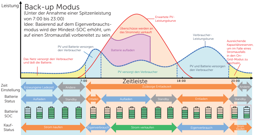
Abbildung 2-27 Backup-Modus
