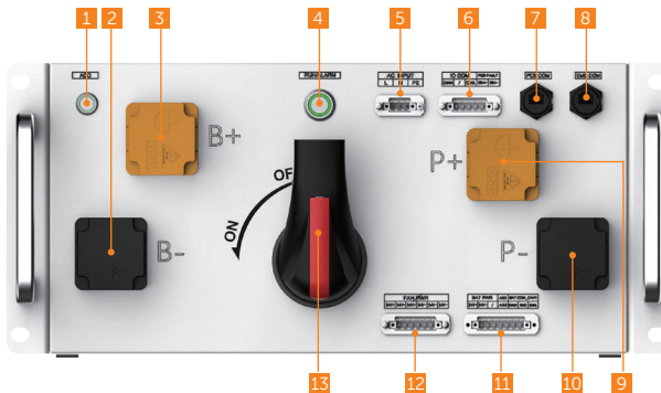
Abbildung 2-8 Frontplatte
