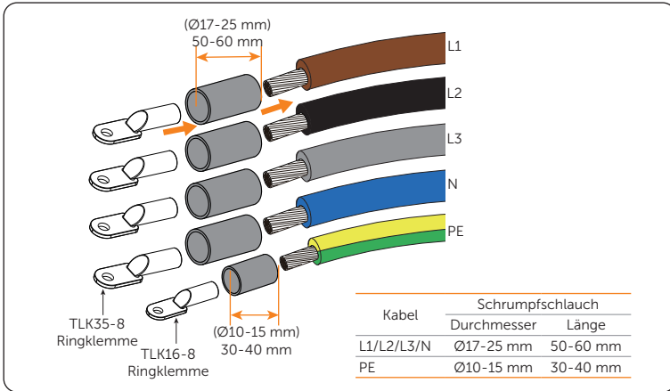
Abbildung 7-71 Schrumpfschläuche schneiden
