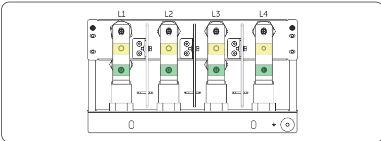
Abbildung 7-76 Anschlussbereich
