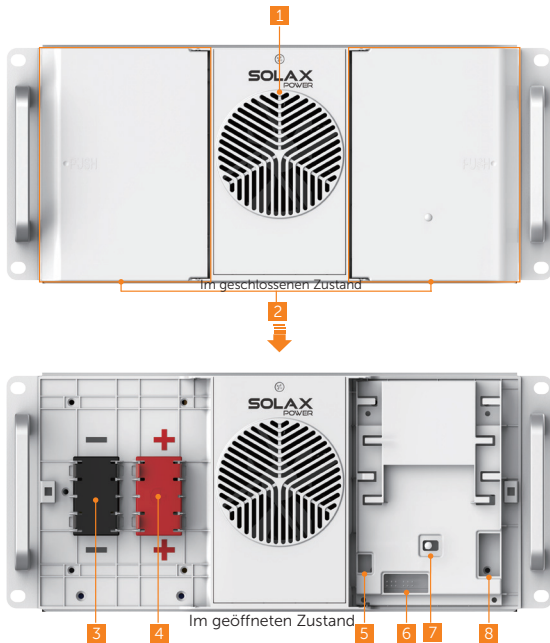
Abbildung 2-9 Frontplatte
