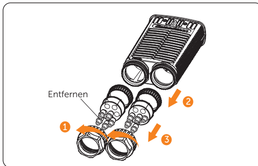
Abbildung 7-8 Den AC-Steckverbinder demontieren
