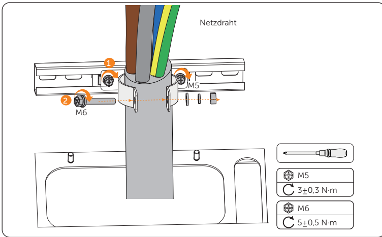
Abbildung 7-79 Schrauben anziehen
