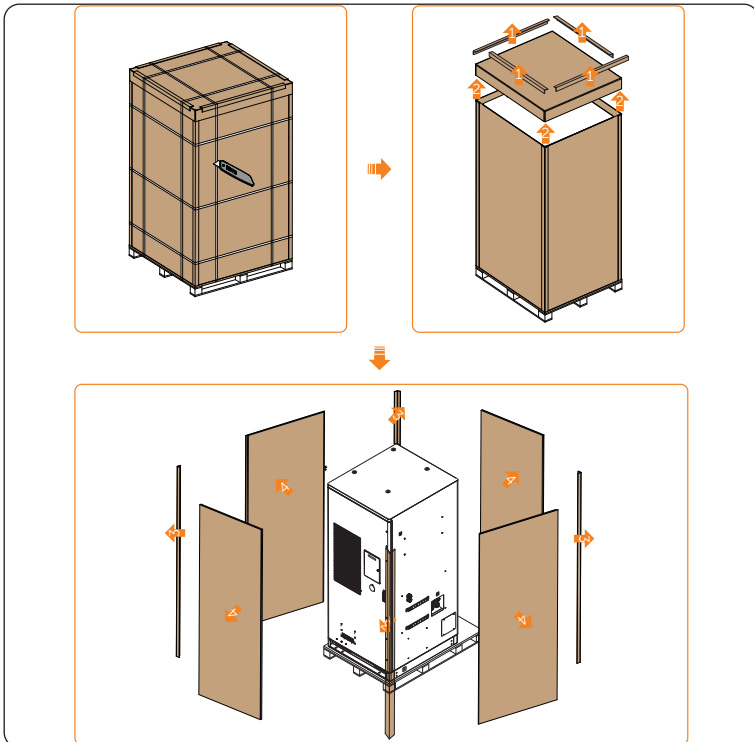
Abbildung 5-1 Auspacken
