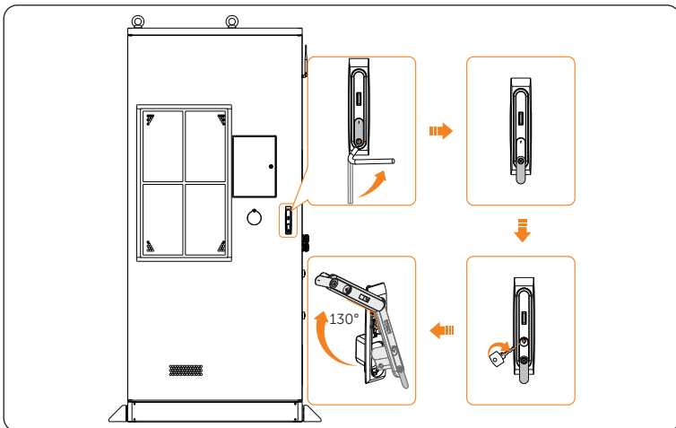
Abbildung 7-61 Vordertür öffnen
