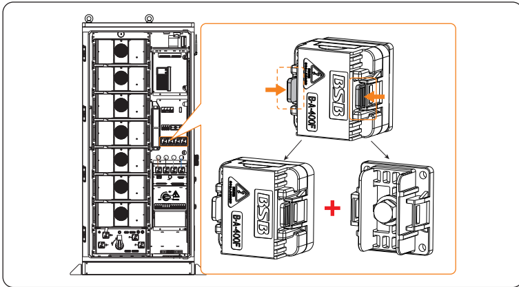
Abbildung 7-66 Abdeckungen herausziehen
