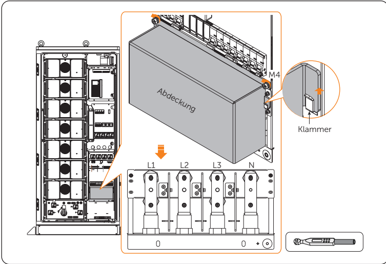
Abbildung 7-75 Abdeckung entfernen
