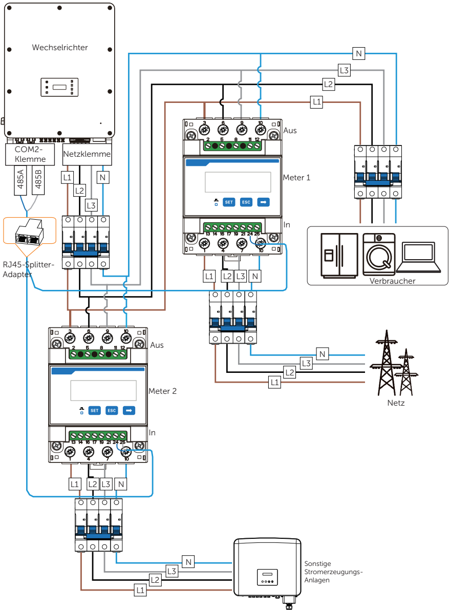
Abbildung 14-26 Anschlussplan von zwei direkt angeschlossenen Metern
