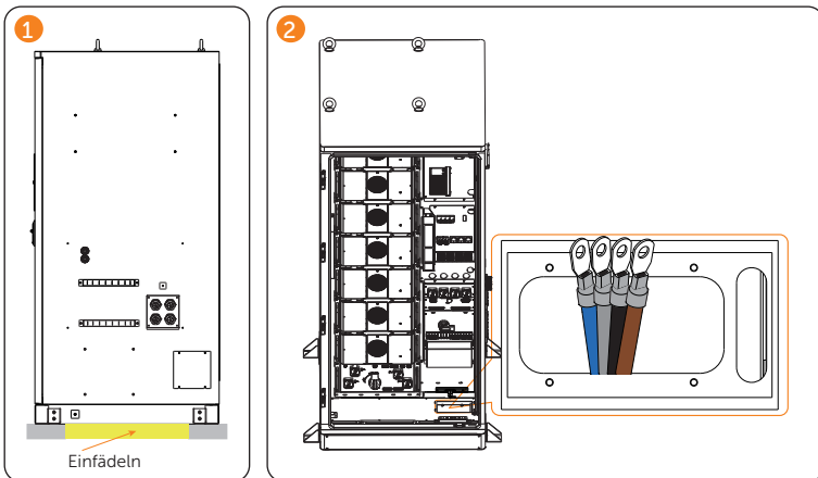
Abbildung 7-63 EPS-Drähte einfädeln
