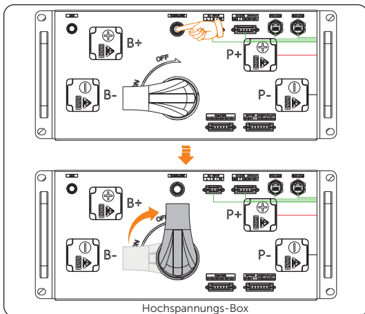
Abbildung 11-6 Hochspannungsbox ausschalten
