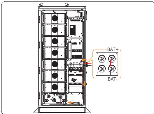
Abbildung 14-41 Einfädelrichtung
