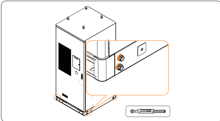
Abbildung 6-10 M12-Schrauben abschrauben
