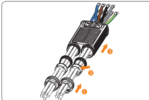
Abbildung 7-9 Kabel durch den AC-Steckverbinder führen
