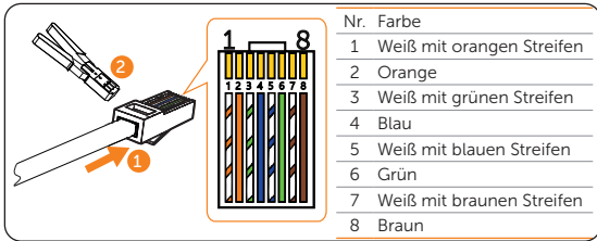
Abbildung 9-20 RJ45 crimpen
