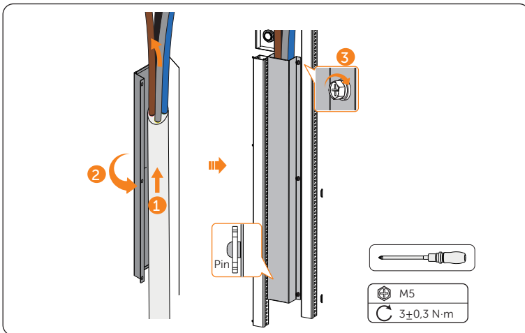
Abbildung 7-65 EPS-Draht einfädeln
