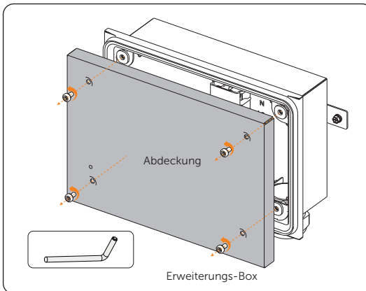
Abbildung 14-74 Gehäusedeckel entfernen
