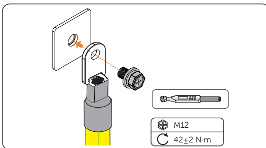
Abbildung 7-6 M12-Schrauben anziehen
