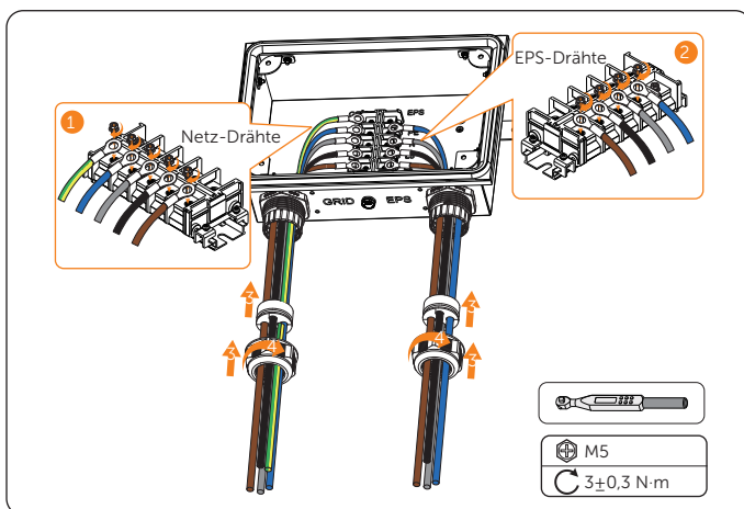
Abbildung 14-80 NETZ- und EPS-Drähte anschließen
