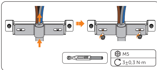
Abbildung 14-53 Netzdräht einfädeln
