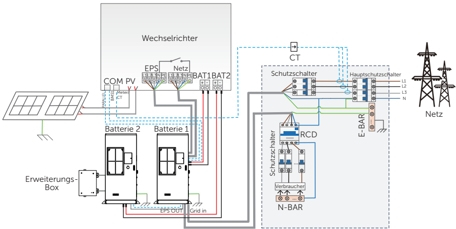
Abbildung 2-35 Vollständiges Verbraucher-Backup für Australien
