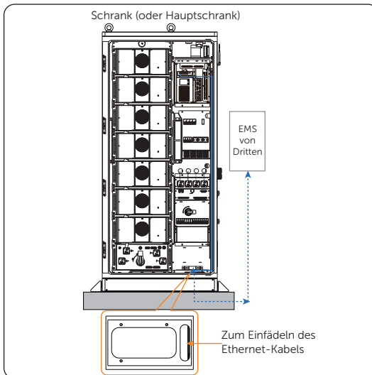
Abbildung 9-24 Ethernet-Kabel einfädeln
