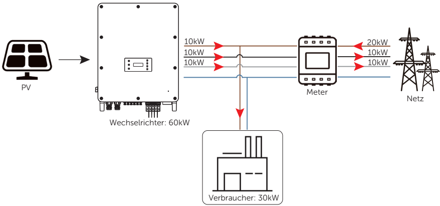
Abbildung 2-30 Null-Einspeisen-Begrenzung mit deaktivierter Phasensymmetrie
