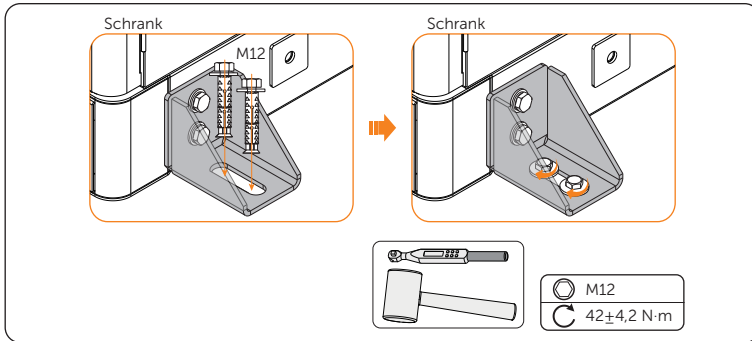
Abbildung 6-14 Spreizdübel anziehen
