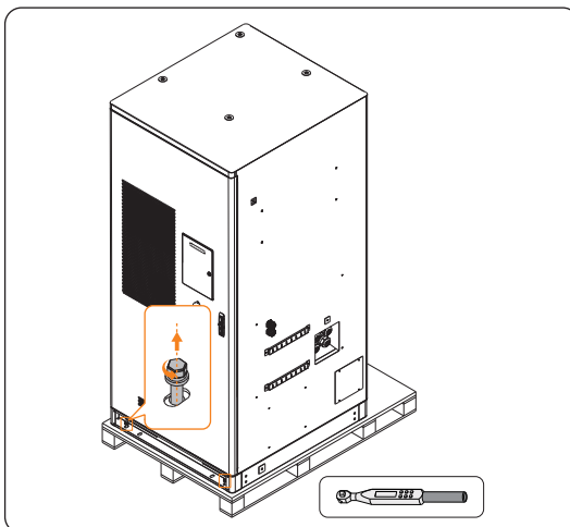
Abbildung 6-2 M12-Schraube abschrauben
