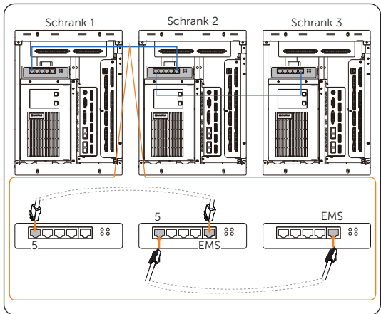
Abbildung 14-100 Ethernet-Kabel anschließen
