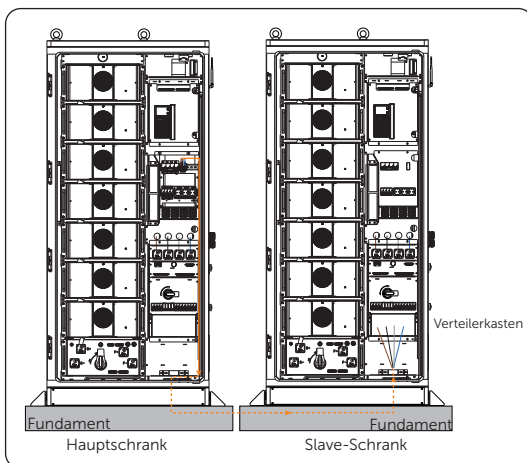
Abbildung 14-51 Kabel einfädeln
