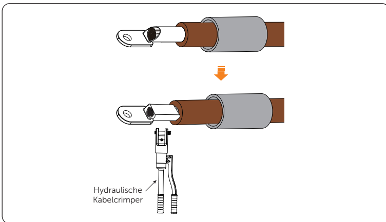
Abbildung 7-72 Crimpen
