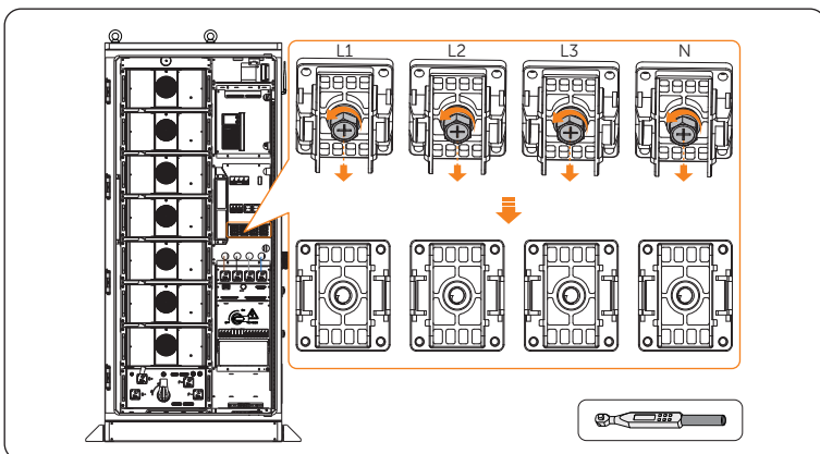
Abbildung 7-67 M8-Schrauben abschrauben
