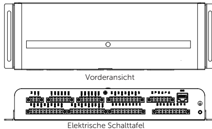
Abbildung 2-11 IO-Modul
