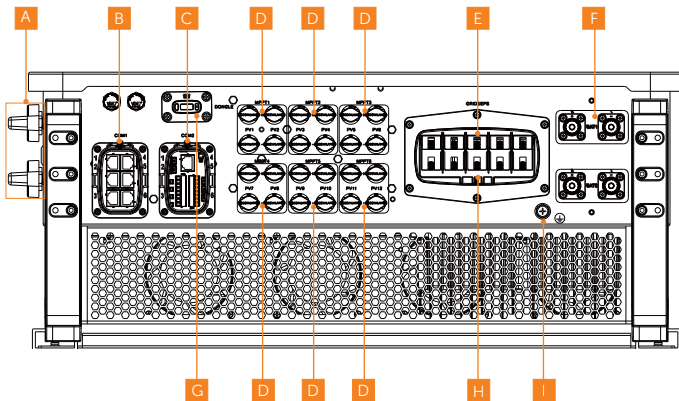
Abbildung 7-7 Klemmen des Wechselrichters
