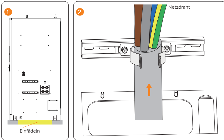
Abbildung 7-77 GRID-Drähte einfädeln
