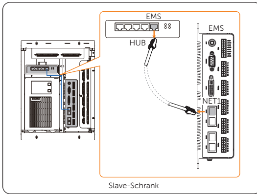
Abbildung 14-65 Kabel ausziehen
