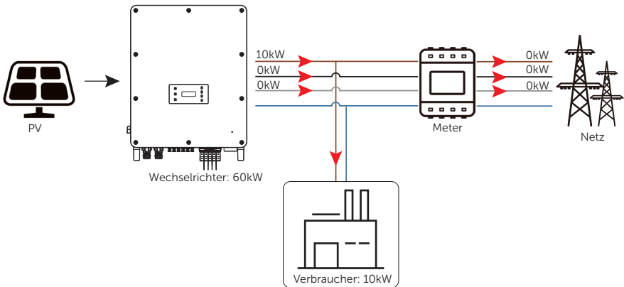
Abbildung 2-31 Null-Einspeisen-Begrenzung mit aktivierter Phasensymmetrie
