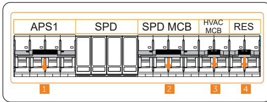
Abbildung 11-9 Schutzschalter herunterklappen
