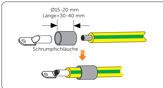
Abbildung 7-3 Schrumpfschläuche schneiden
