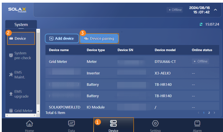
Abbildung 14-87 Gerät koppeln
