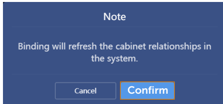
Abbildung 14-89 Kopplung bestätigen
