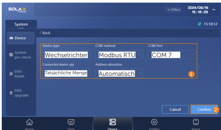
Abbildung 14-109 Parameter einstellen
