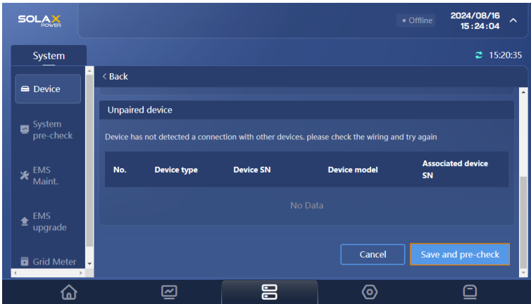
Abbildung 14-111 Kopplung speichern
