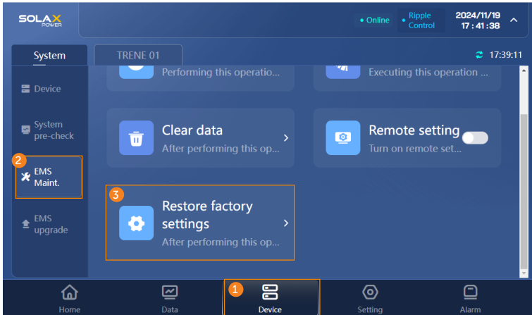
Abbildung 14-107 Werkseinstellungen zurücksetzen
