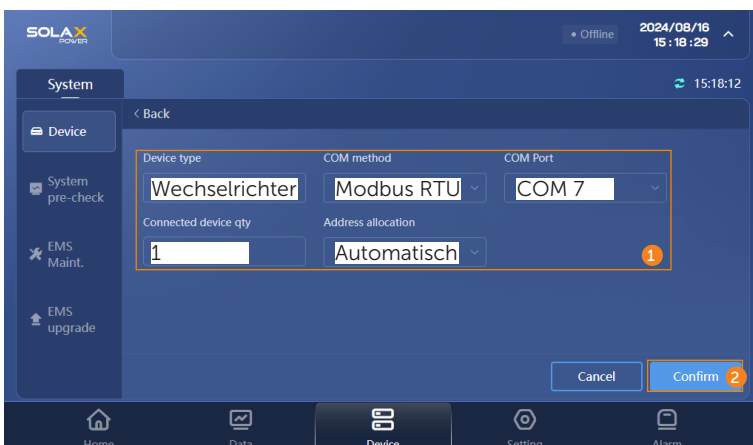
Abbildung 9-12 Parameter einstellen
