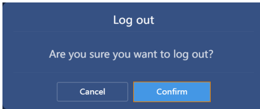
Abbildung 9-9 Abmelden
