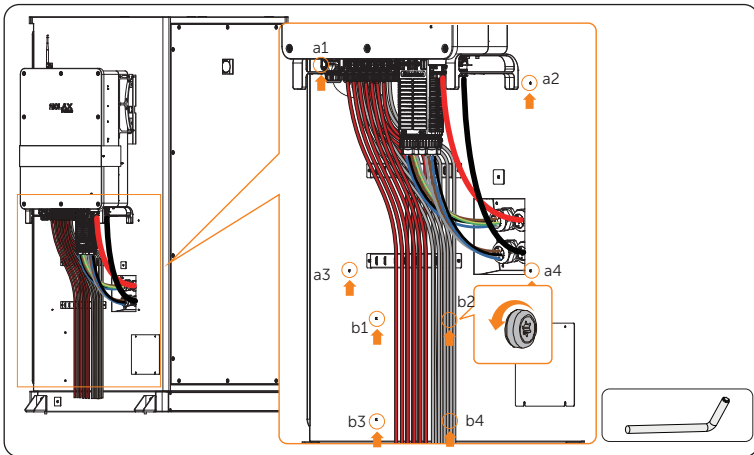
Abbildung 7-83 M6-Schrauben herausdrehen
