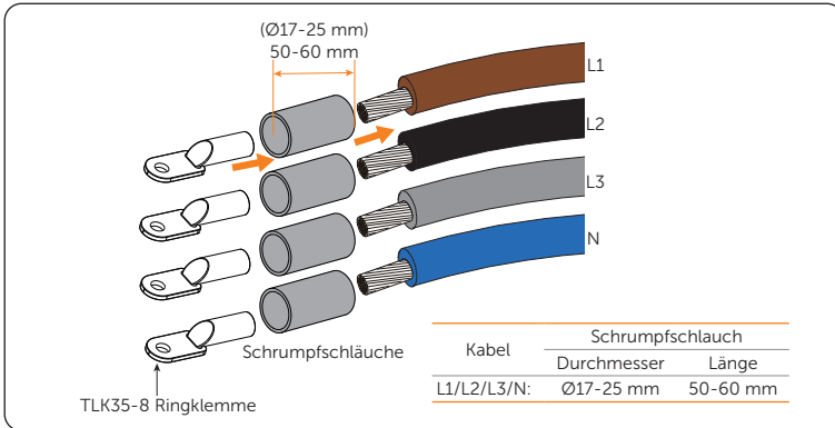
Abbildung 7-58 Drähte stecken
