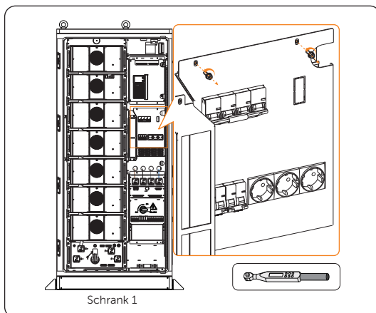
Abbildung 14-46 Abdeckung entfernen
