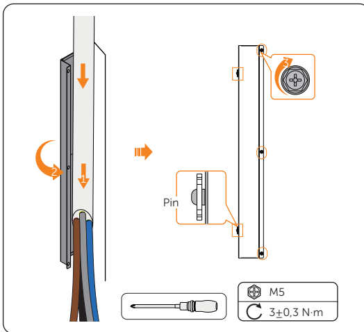
Abbildung 14-49 EPS-Draht einfädeln
