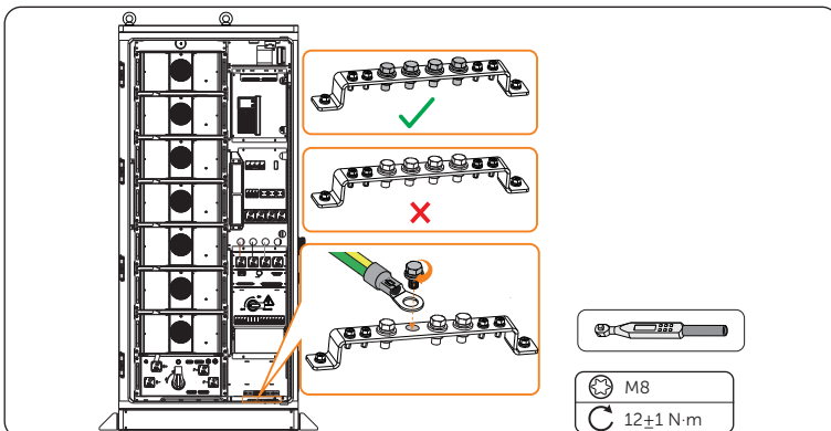
Abbildung 7-80 PE-Draht anschließen
