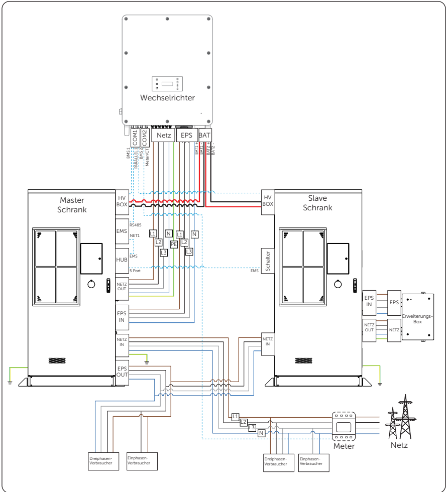
Abbildung 14-31 System-Schaltplan
