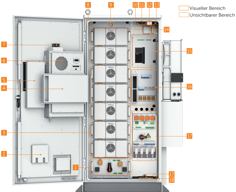
Abbildung 2-5 Teile-Beschreibung (im geöffneten Zustand)
