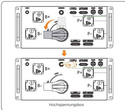
Abbildung 8-8 Hochspannungskasten starten
