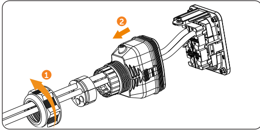
Abbildung 14-39 Netzwerkkabel entfernen
