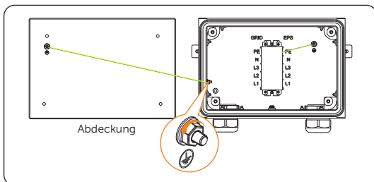
Abbildung 14-75 M5-Mutter abschrauben
