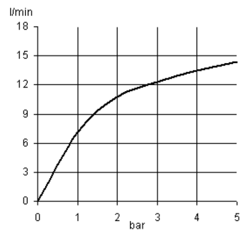
Durchflussdiagramm
