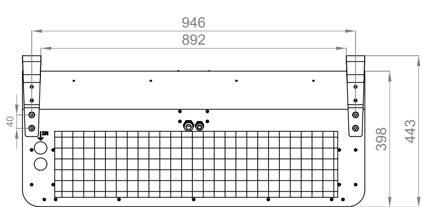
Unteransicht
