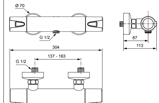
Maßzeichnung
