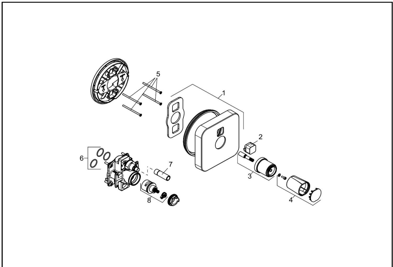
V4TFM1E Farbset indiv.3.0 TipTec Mischer für 1 Verbraucher eckig f.VIGUPK verchr. VIG Finish indiv. 3.0 TipTec mixer 1 user quare f. VIGUPK chromed VIGOUR
