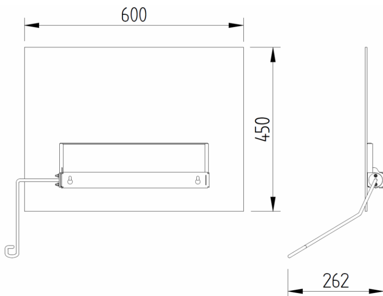
Technische Zeichnung (Ausführung Rechts)
