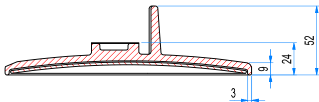
A-A (1:2)
