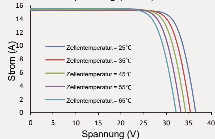
Strom-Spannung (450W)
