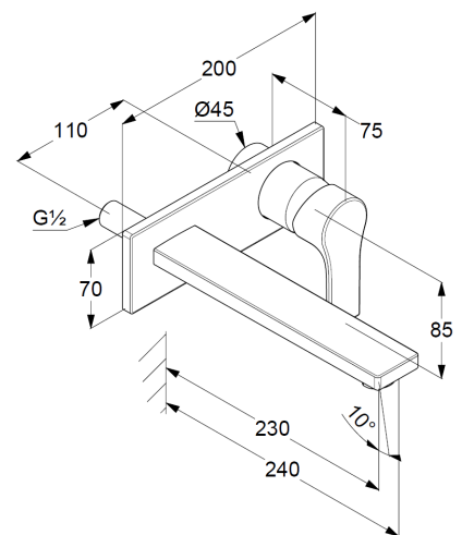
Maßzeichnung/ Dimensional drawing
