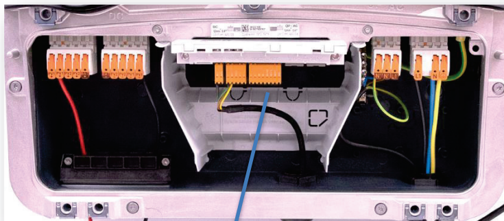
Abbildung 2: 16- poliger Stecker bei GEN24 Plus Wechselrichtern. Pin IO 0-3 und GND zur Relaisansteuerung verwenden.
