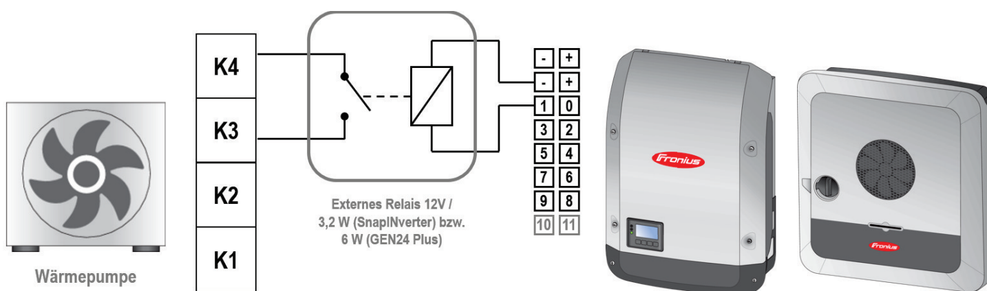
Abbildung 1: Anschlussschema des externen Relais für die Smart Grid Ready Ansteuerung
